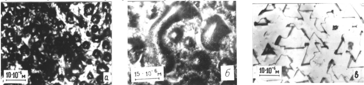
Рис. 3.3. Морфологія поверхні плівок \text{PbSe} , осаджених: а – із наважки стехіометричного складу; б – при пересиченні пари свинцем; в – при пересиченні пари телуром [10].
