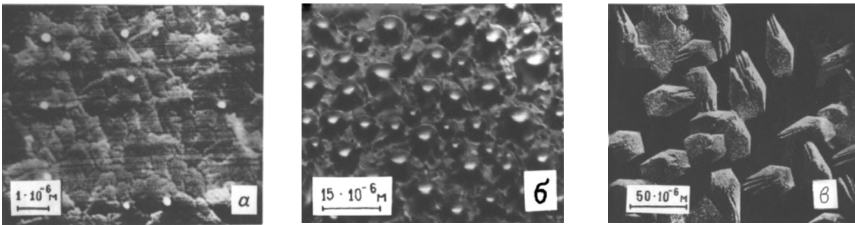
Рис. 3.2. Морфологія поверхні плівок \text{PbTe} , осаджених: а – із наважки стехіометричного складу; б – при пересиченні пари свинцем; в – при пересиченні пари телуром [10].
