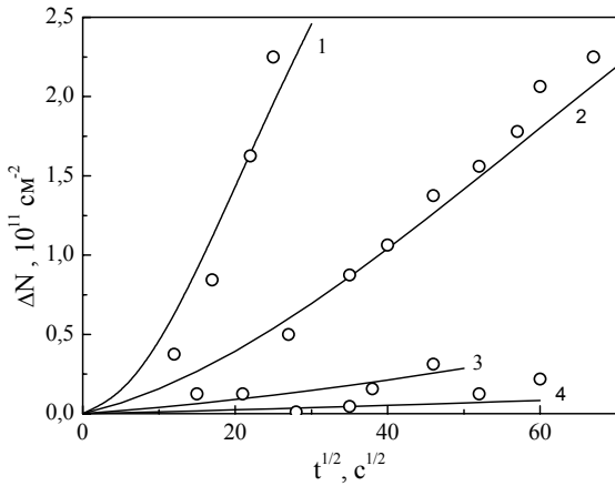
Рис. 5.1. Зменшення поверхневої концентрації електронів у плівці n-PbTe при різних тисках кисню: 1 – 1,333 \cdot 10^{-4} , 2 – 1,333 \cdot 10^{-5} , 3 – 1,333 \cdot 10^{-6} , 4 – 1,333 \cdot 10^{-7} Па; о – експериментальні результати, суцільні лінії – розрахункові криві. Вихідна кон-центрація електронів n_0 = 1,6 \cdot 10^{17} \text{ см}^{-3} [84].
