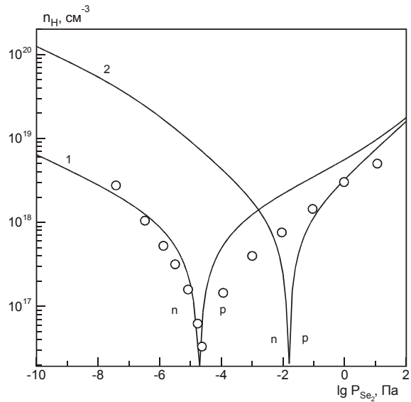
Рис. 4.4. Залежність концентрації n_H від тиску пари селену при врахуванні наявності кисню у плівках PbSe. T_e = 820K , T_s = 700K , P_{O_2} = 10^{-4} Pa . ○ – експериментальні результати; 1 і 2 – розрахункові криві відповідно із врахуванням і без врахування кисню [22].
