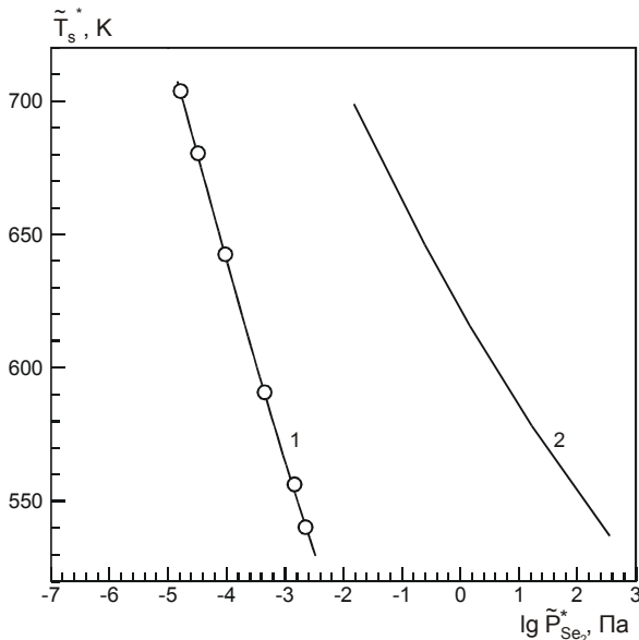
Рис. 4.1. Залежність температури \tilde{T}_s^* термодинамічної n-p – інверсії від парціального тиску пари селену в плівках PbSe. T_e = 820K , P_{O_2} = 10^{-4} Pa . \circ – експериментальні результати; 1 і 2 – розрахункові криві відповідно із врахуванням і без врахування кисню [22, 78].
