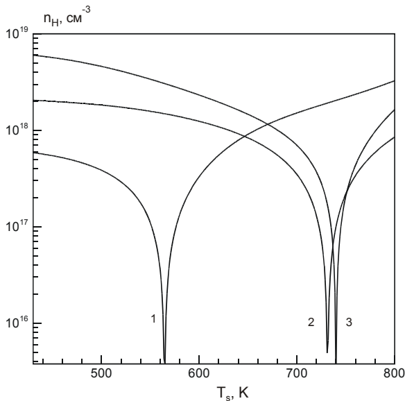
Рис. 4.3. Залежність концентрації дефектів [O_i^-] , [V_{Pb}^-] від температури осадження при врахуванні наявності кисню у плівках PbSe. T_e = 820K , P_{Se_2} = 10^{-2} Pa , P_{O_2} = 10^{-4} Pa . (1) та (2) – концентрації [O_i^-] та [V_{Pb}^-] відповідно [22].
