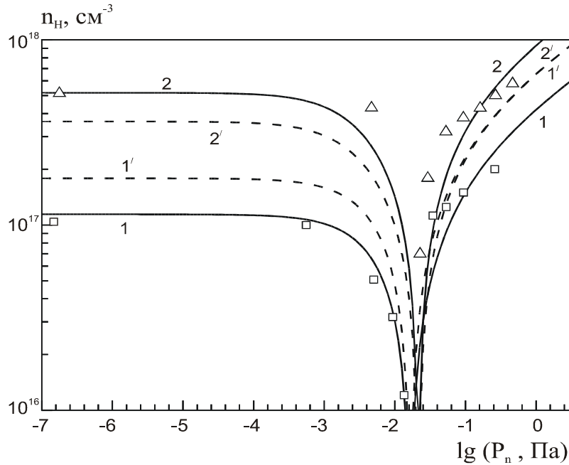
Рис. 2.1. Залежності концентрації носіїв струму n_H у плівках PbTe від номінального тиску пари телуру ( T_s = 653\text{K} , T_e = 833\text{K} ); підкладки:
