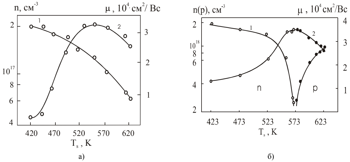
Рис. 3.1. Залежність концентрації n (1) і рухливості \mu (2) носіїв струму від температури осадження T_s (метод гарячої стінки; підкладка – сколи (111) \text{BaF}_2 ; T_c = 820\text{K} ; T_w = 850\text{K} : (а) – для плівок \text{PbTe} , P_{\text{Te}_2} = 1,3 \cdot 10^{-2} \text{Па} , (б) – для плівок \text{PbSe} , P_{\text{Se}_2} = 10^{-3} \text{Па} [10].
