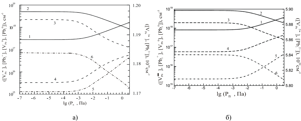
Рис. 2.2. Залежності розрахованих значень концентрацій дефектів у плівках PbTe, вирощених на підкладках BaF 2 (а) і NaCl (б) від номінального тиску пари телуру ( T_s = 653\text{K} , T_e = 833\text{K} ); 1 і 2 – однозарядні дефекти [V_{Pb}^-] і [Pb_i^+] , 3 і 4 – двократно заряджені дефекти [V_{Pb}^{2-}] і [Pb_i^{2+}] , 5 і 6 – електронейтральні дефекти [V_{Pb}^0] і [Pb_i^0] відповідно [18].
