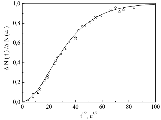
Рис. 5.2. Зменшення приведеної поверхневої концентрації електронів в плівках n-PbTe до рівня, що відповідає власній концентрації при тиску кисню 1,333 \cdot 10^{-4} Па; концентрація електронів n_0 : 1-4 – 5 \cdot 10^{16} ; 8 \cdot 10^{16} ; 9 \cdot 10^{17} ; 1,5 \cdot 10^{18} \text{ см}^{-3} ; Δ-1, □-2, ×-3, о-4. Суцільна лінія – розрахункова крива [84].
